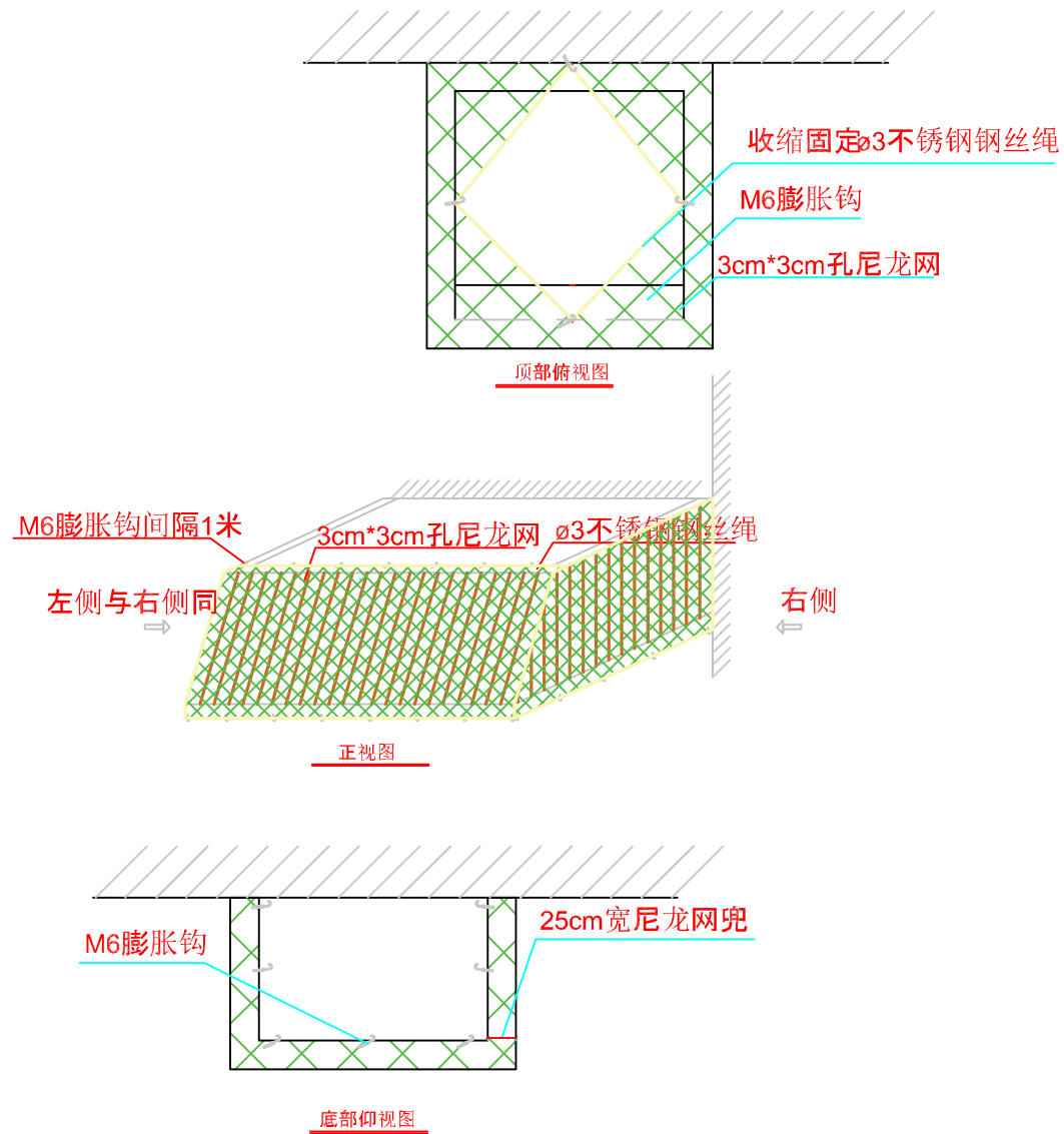
防护网整体示意图
